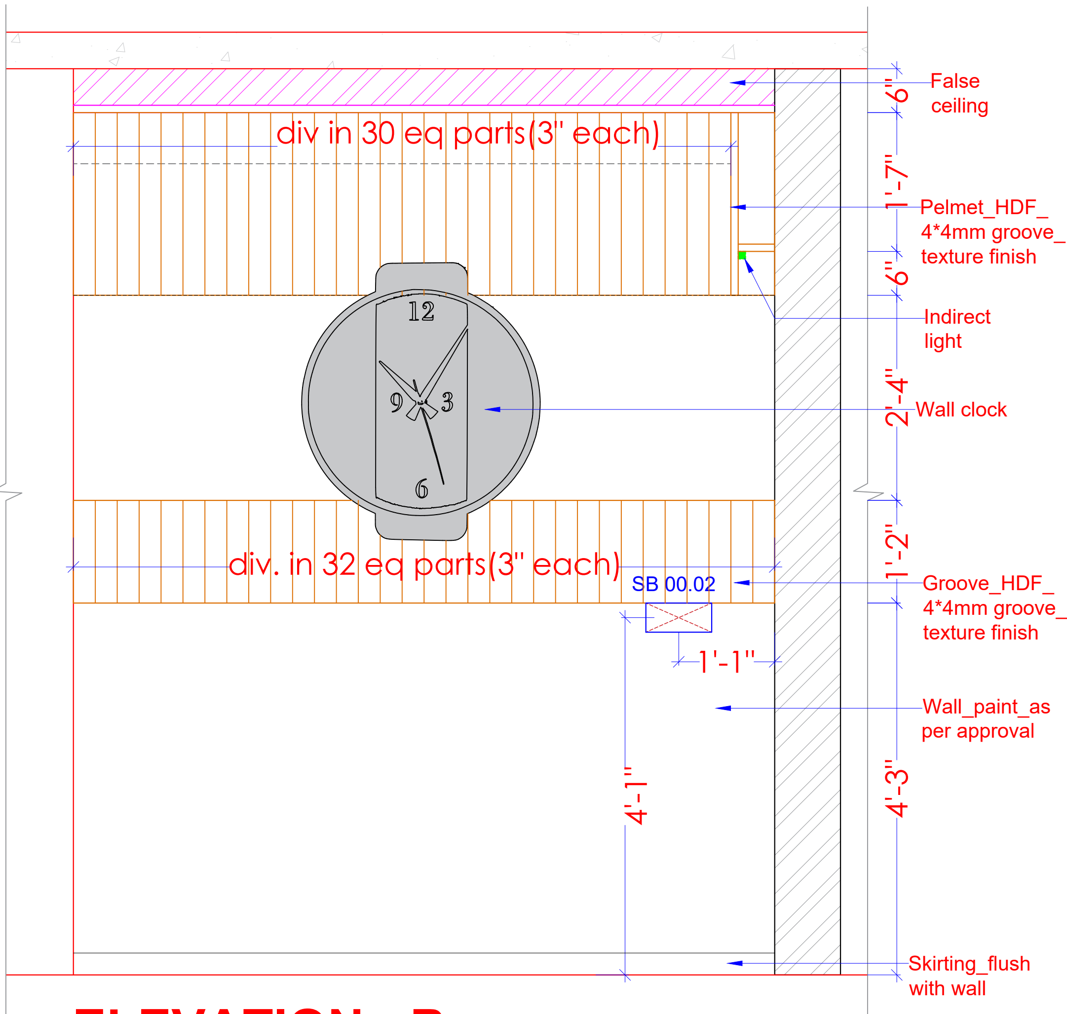
ELEVATION - B
